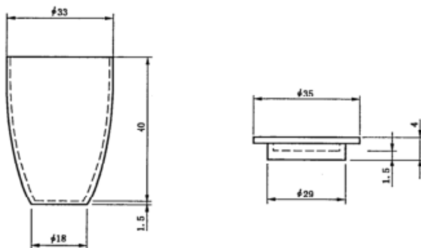
图 3 挥发分坩埚
