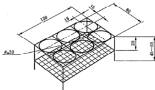
图4 坩埚架
