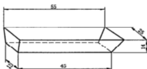
图 2 灰皿
